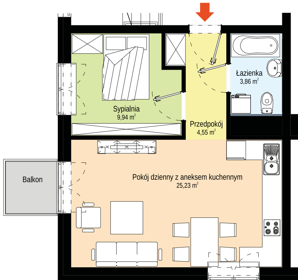
Okno tylko w mieszkaniach D.1.2, D.2.2, D.3.2, D.4.2, D.5.2, D.6.2.
